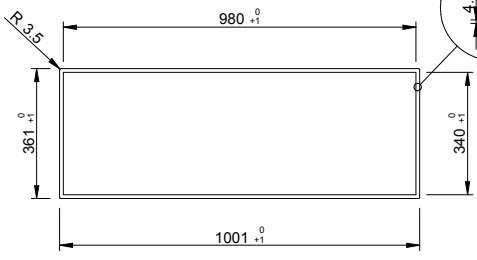
POSITIE AFDICHTINGSMIDDEL IN DE FILOTOP-VERSIE
