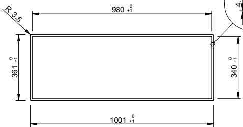
POSITIE AFDICHTINGSMIDDEL IN DE FILOTOP-VERSIE
