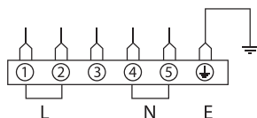
Схема підключення
