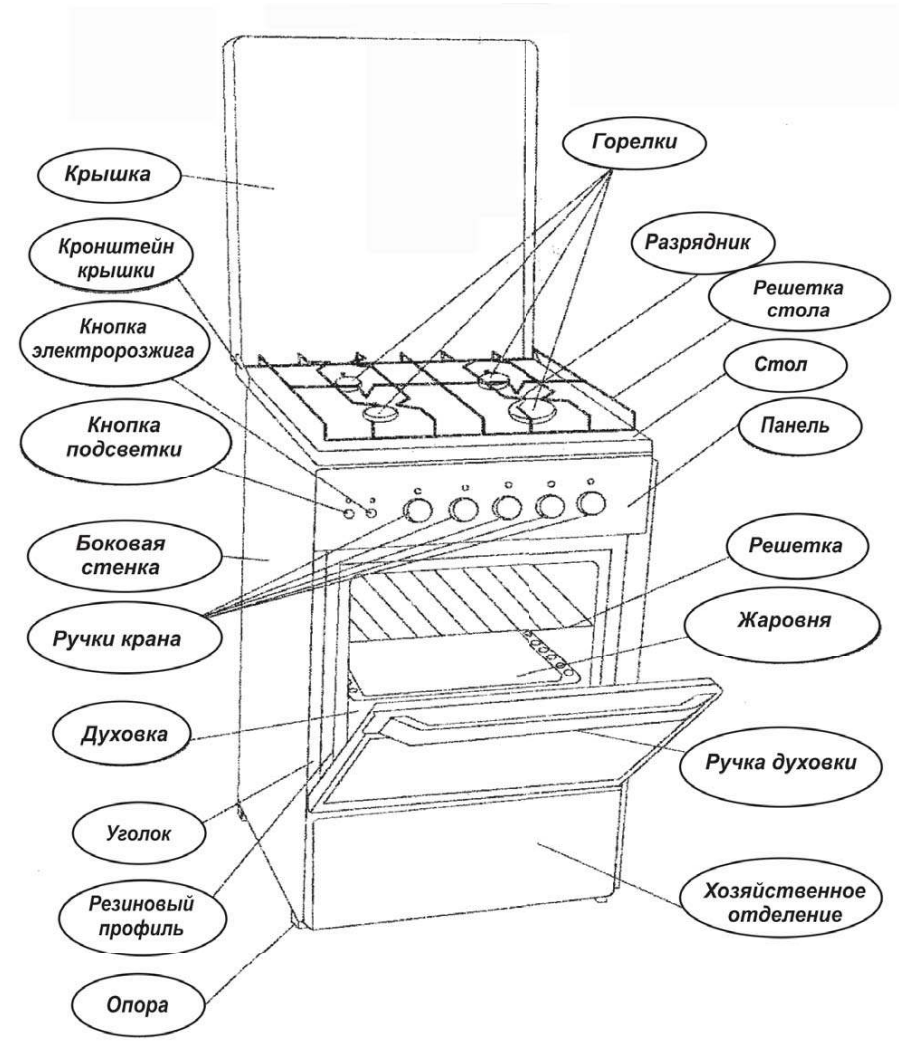
Рис. 1 Устройство плиты
