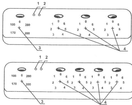
Рис. 2. Панель электроплиты (трех и четырехконфорочная)
