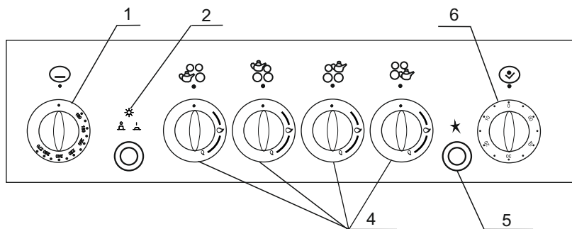
Панель управления плит моделей 5040.36г, 5040.44г
