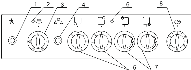
Панель управления плиты модели 5422.00гэ
