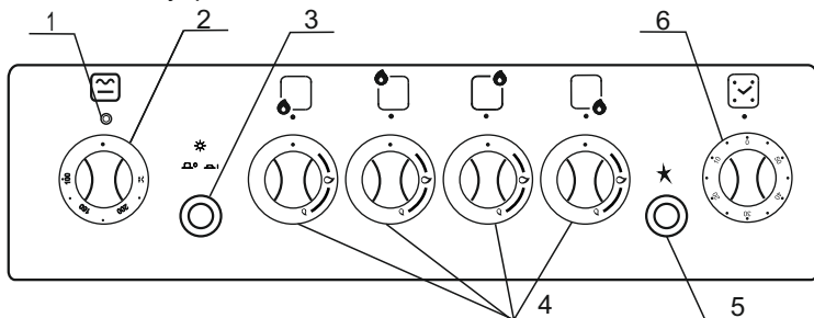
Панель управления плиты модели 5040.20гэ, 5040.30гэ
