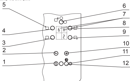
рис. 5. Сенсорная панель управления
