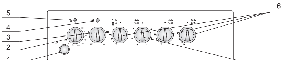
рис. 11. Панель плиты без таймера
