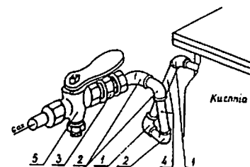
Przekłady gazowego do kuchni: a) - na rurociągu poziomym b) - na rurociągu pionowym 1 - trójnik do sprawdzania instalacji 2 - kurek odcinający 3 - dwuzłazka do podłączenia kuchni.
