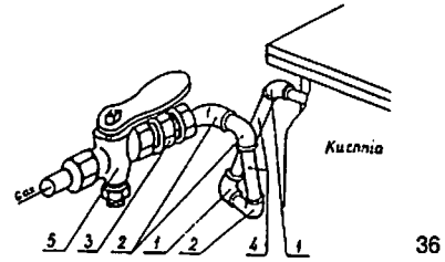
Przykłady gazowego do kuchni: a) - na rurociągu poziomym b) - na rurociągu pionowym 1 - trójnik do sprawdzania instalacji 2 - kurek odcinający 3 - dwuzłazka do podłączenia kuchni.
