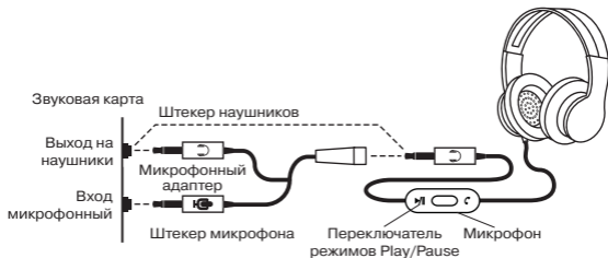
Рис. 1. Схема подключения
