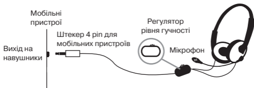
Мал. 1. Схема підключення
