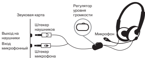
Рис. 1. Схема подключения
