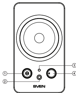
Рис. 1. Панель управления
