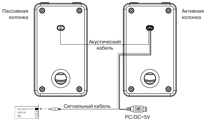
Рис. 2. Схема подключения
