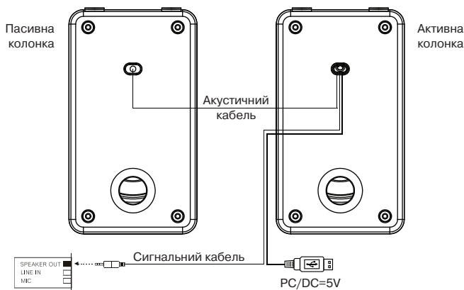
Мал. 2. Схема підключення
