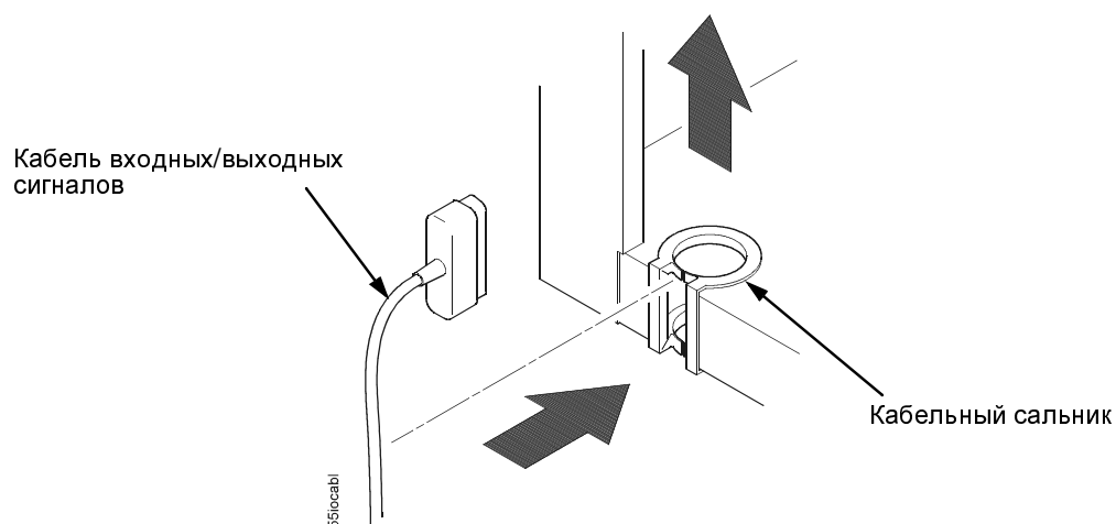
Рисунок 14. Прокладка кабеля входных/выходных сигналов
