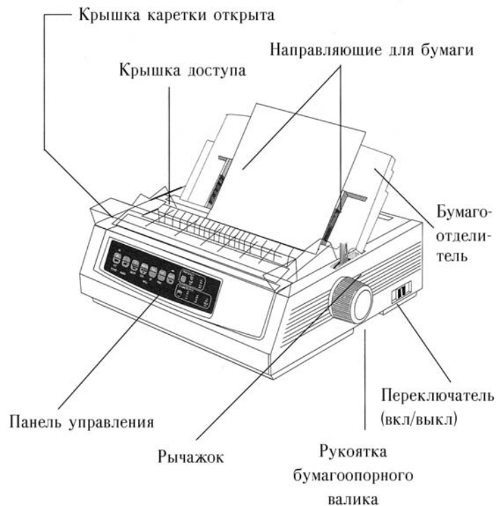
Установка для подачи одиночных листов
