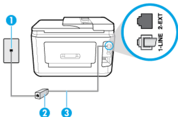
Рисунок 5-2 Вид принтера сзади
