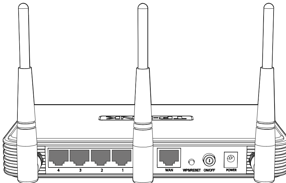
Рис. 1-2 Задняя панель
