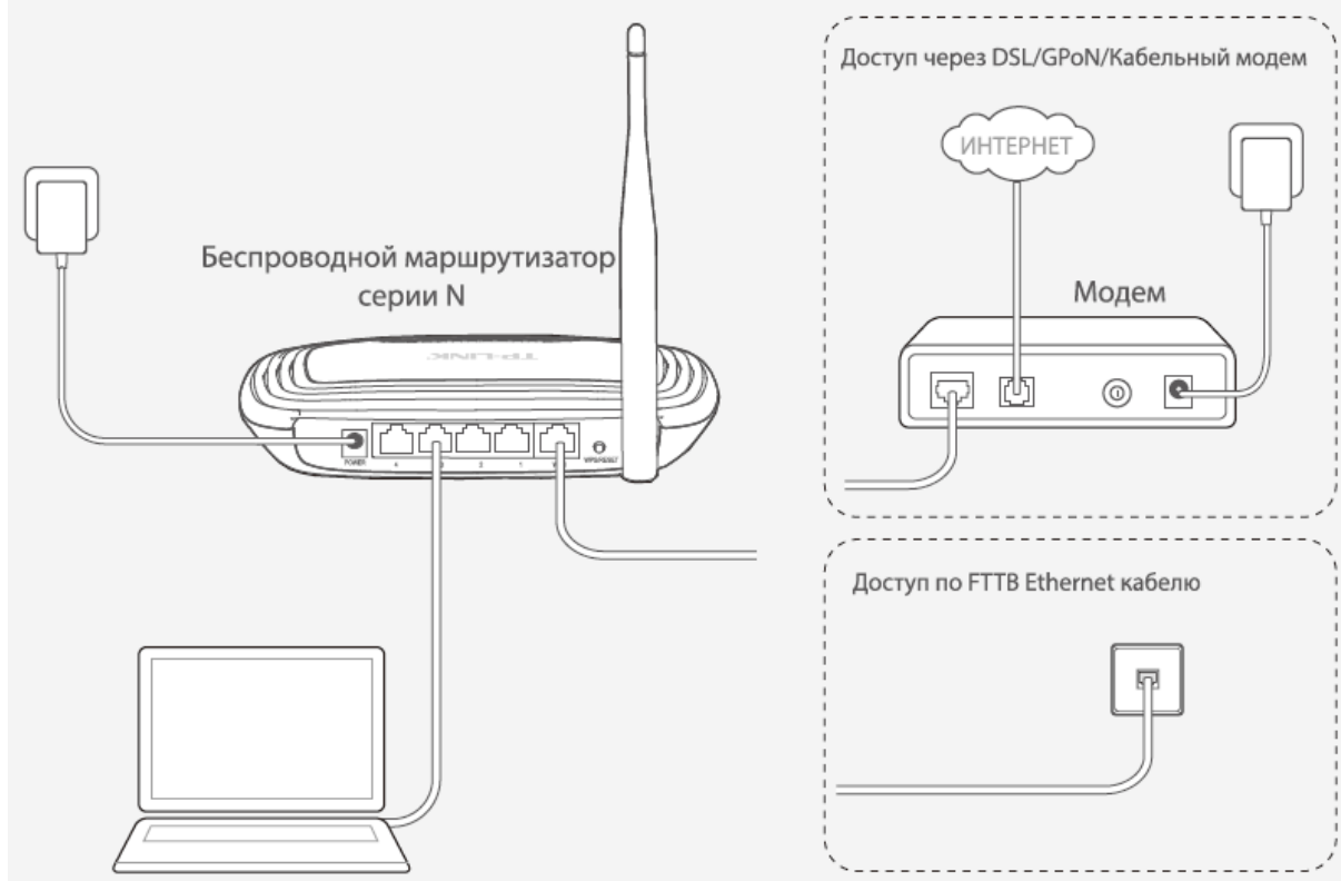
Рис 2-1 Установка аппаратной части маршрутизатора TL-WR740N
