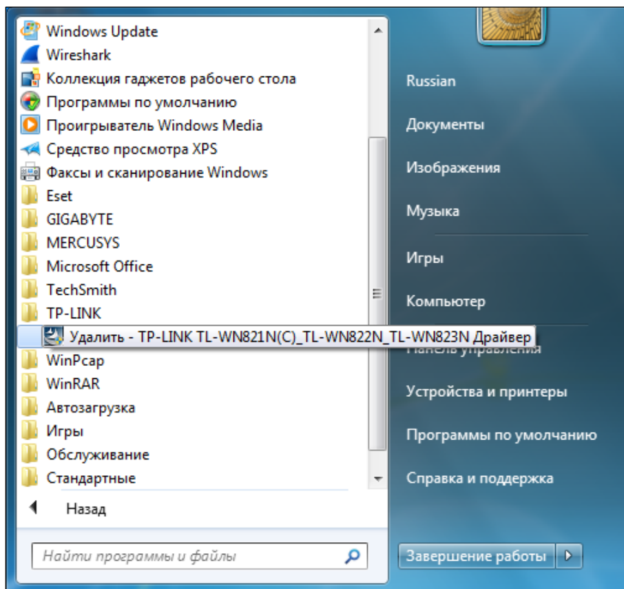
Рис. 6-4 Удаление драйверов
