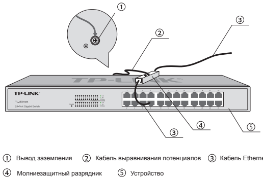
Рисунок 3-4 Выравнивание потенциалов
