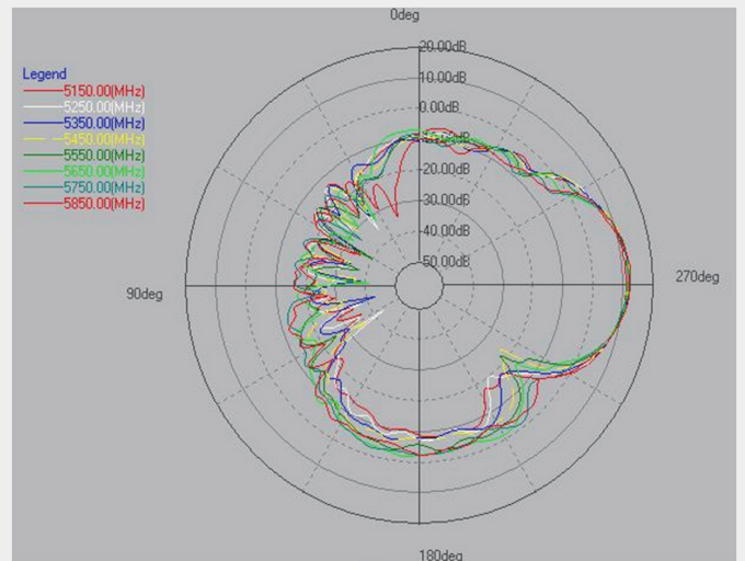
5G (PHI=90)
