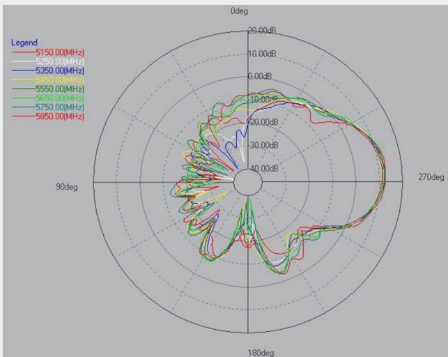
5G (PHI=0)
