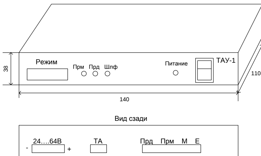
Рисунок 1 – Внешний вид ТАУ-1
