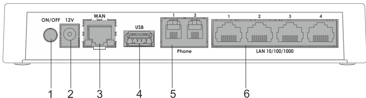
Рисунок 6 – Внешний вид задней панели RG-4402G-W
