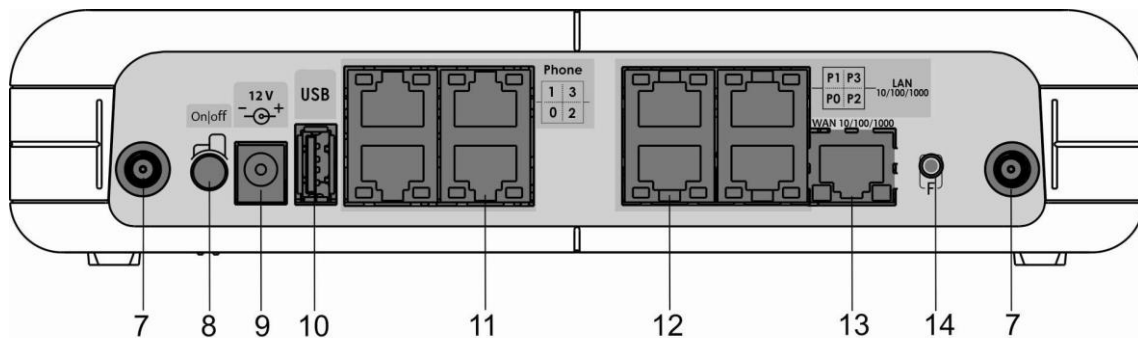
Рисунок 5 – Внешний вид задней панели RG-2404G-W
