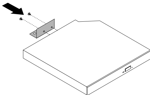
Рис. 21. Установка металлической пластины внешнего дисковод оптических дисков
