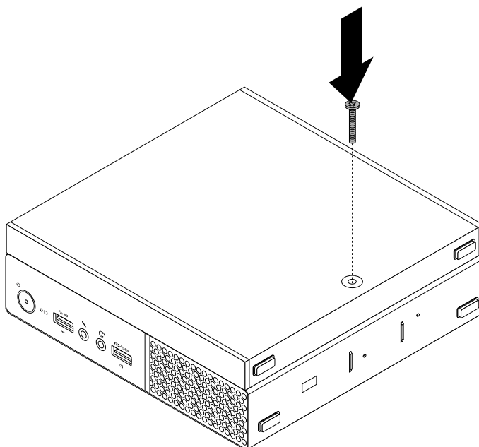
Рис. 25. Установка винта корпуса внешнего дисковод для оптических дисков
