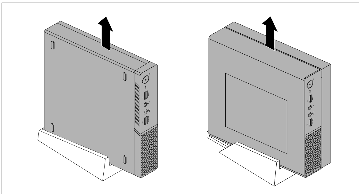
Рис. 12. Снятие компьютера с вертикальной подставки
