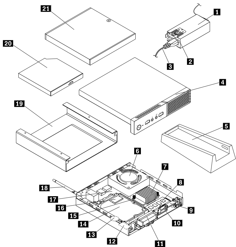
Рис. 3. Компоненты компьютера
