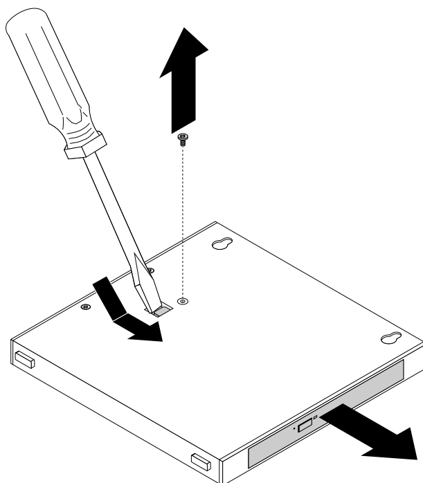
Рис. 19. Извлечение внешнего дисковод для оптических дисков из корпуса
