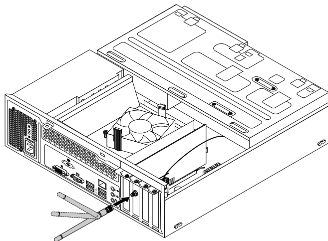
Рис. 50. Установка задней антенны WiFi
