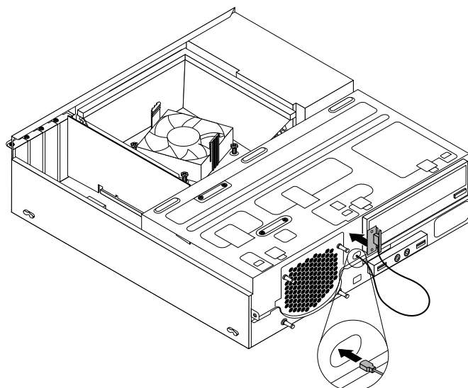
Рис. 53. Установка передней антенны WiFi
