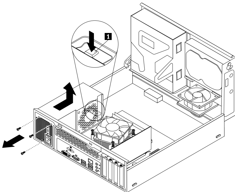
Рис. 31. Как извлечь блок питания
