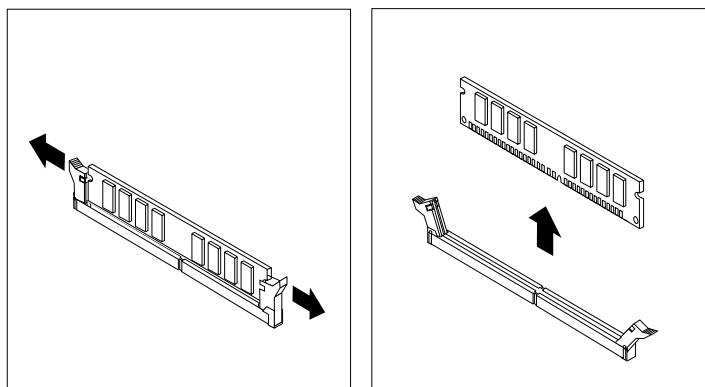
Рис. 15. Как снять модуль памяти
