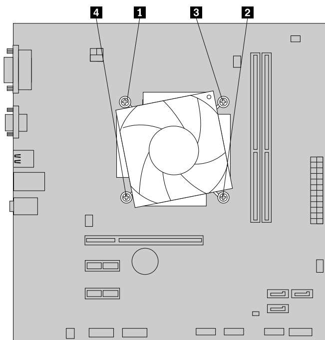
Рис. 35. Как снять блок радиатора и вентилятора
