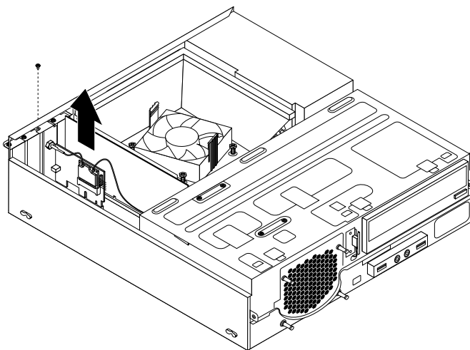
Рис. 43. Извлечение карты контроллера WiFi
