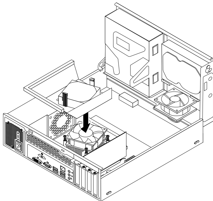
Рис. 33. Установка канала вентилятора радиатора
