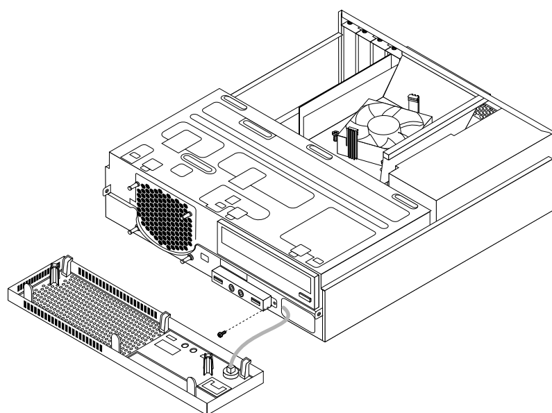
Рис. 42. Как снять передний блок аудиоразъемов и USB
