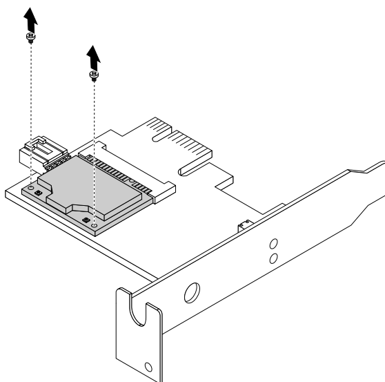
Рис. 45. Снятие винтов для крепления модуля карты WiFi
