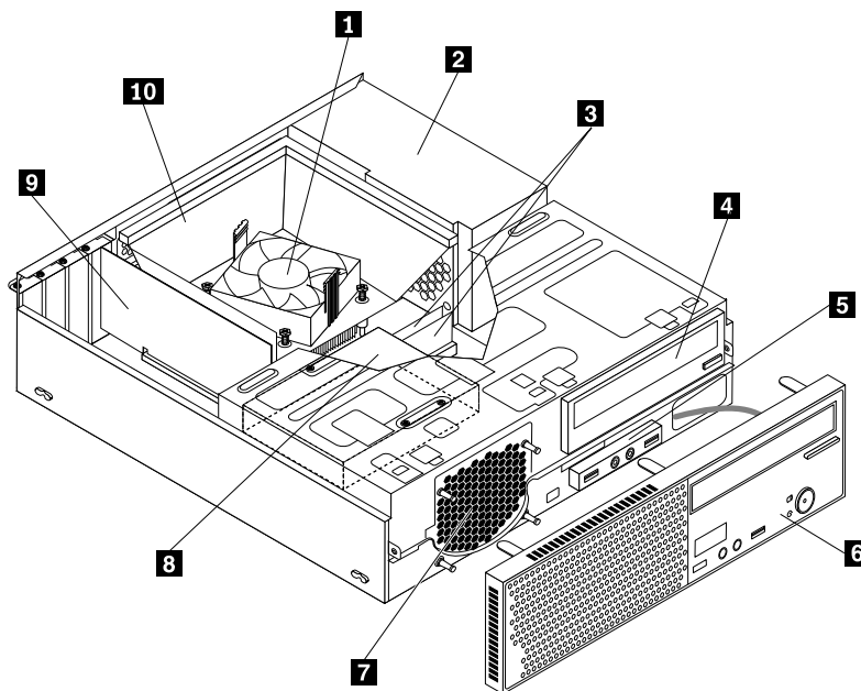
Рис. 3. Расположение компонентов
