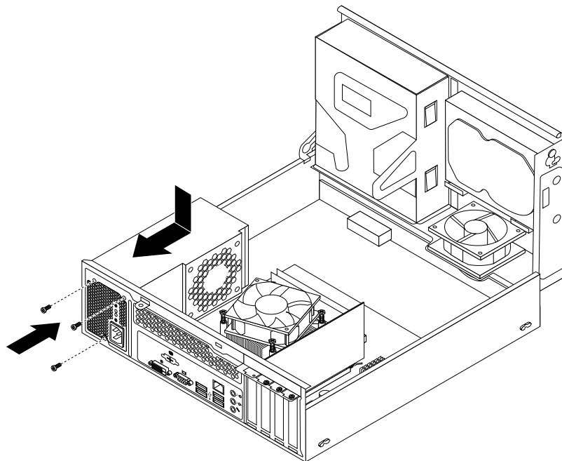
Рис. 32. Установка блока питания
