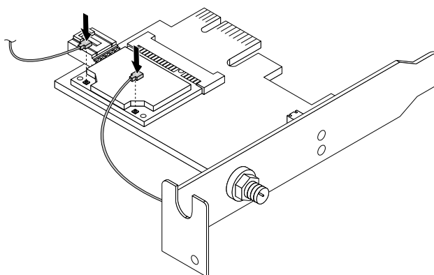
Рис. 48. Подключение кабелей антенн WiFi
