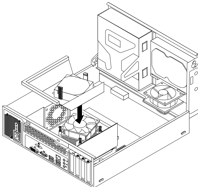
Рис. 36. Установка канала вентилятора радиатора
