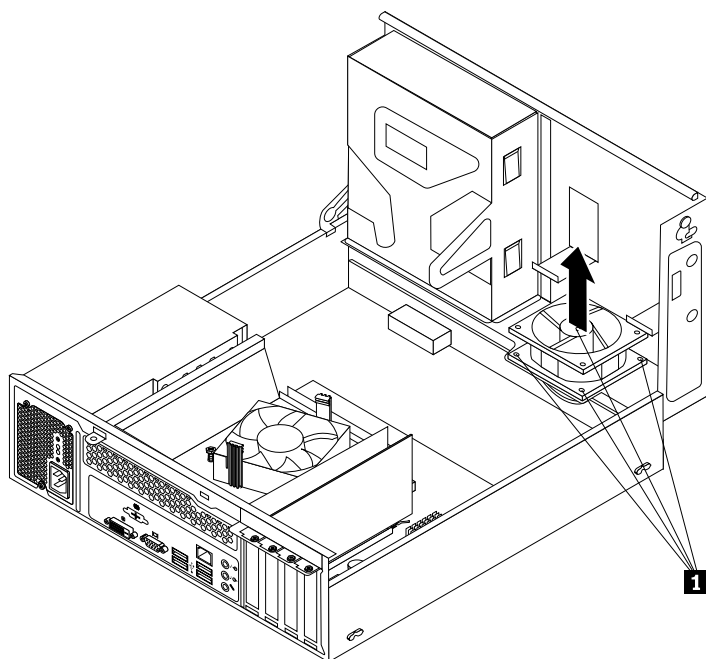
Рис. 40. Извлечение блока вентилятора компьютера
