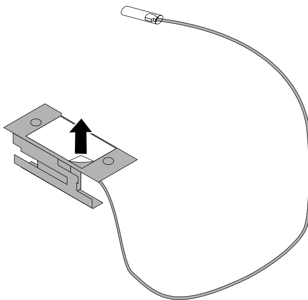
Рис. 52. Снятие бумаги, защищающей клейкий материал
