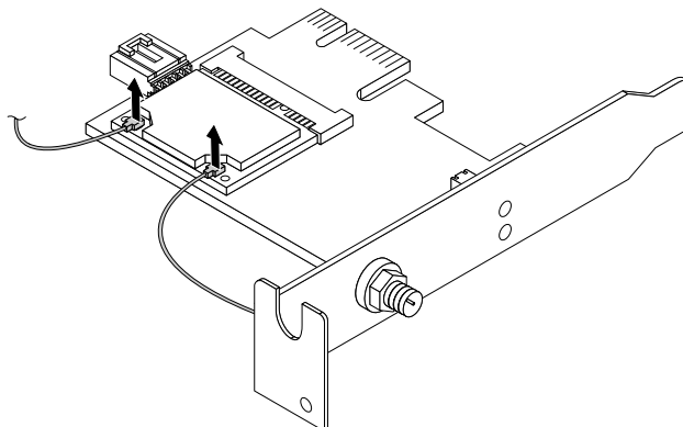
Рис. 44. Отключение кабелей антенн WiFi
