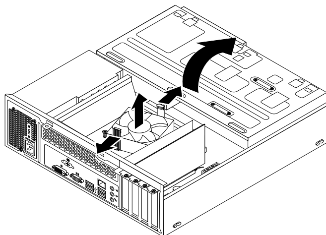
Рис. 34. Как снять канал вентилятора радиатора
