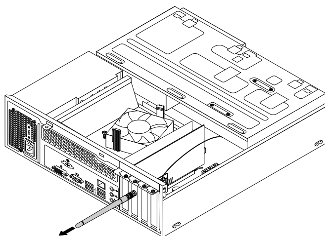
Рис. 51. Снятие задней антенны WiFi
