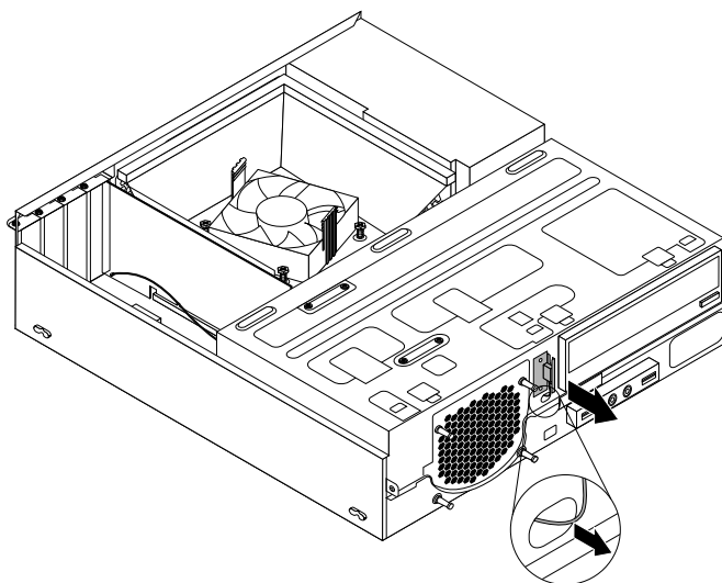
Рис. 54. Снятие передней антенны WiFi
