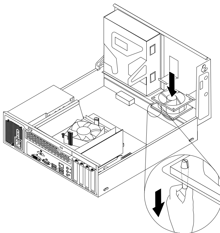
Рис. 41. Установка блока вентилятора компьютера
