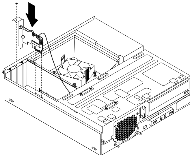
Рис. 49. Установка карты контроллера WiFi
