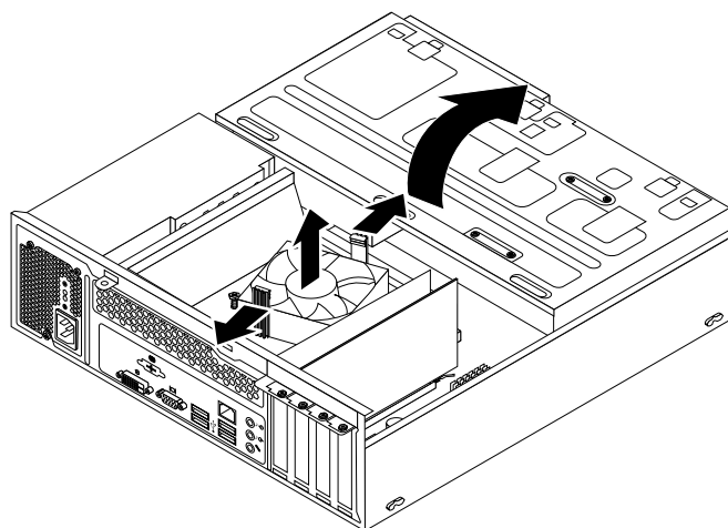
Рис. 30. Как снять канал вентилятора радиатора
