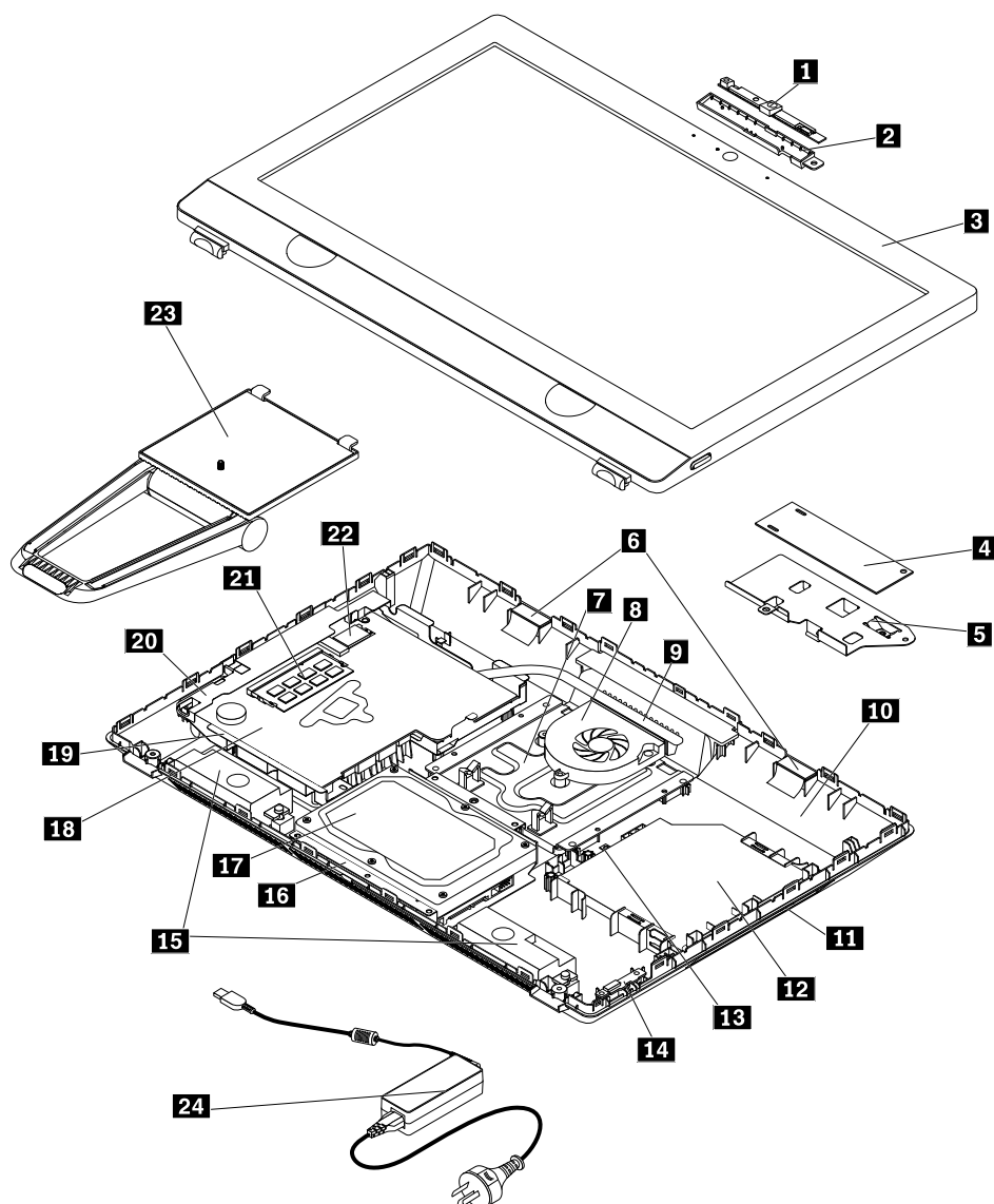
Рис. 3. Компоненты компьютера
