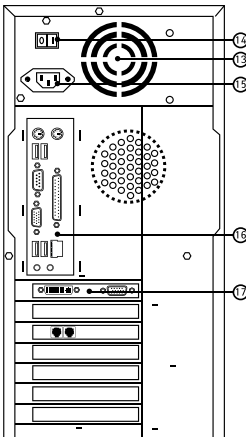
Задняя панель
