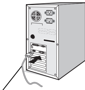
Кабель DisplayPort Рисунок A.4
