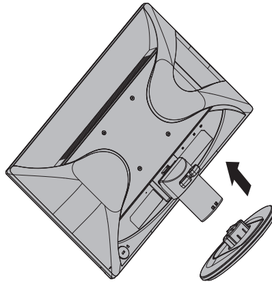
Рис. 3-2 Крепление подставки
