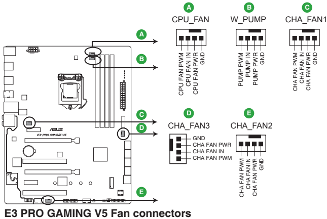
E3 PRO GAMING V5 Fan connectors
