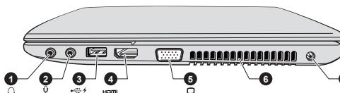
Рисунок 2-3 Правая сторона компьютера
