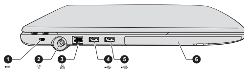
Рисунок 3-2 Левая сторона компьютера
