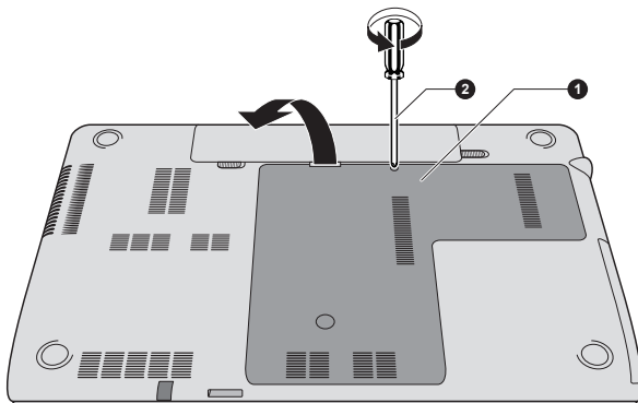
Рисунок 4-13 Снятие крышки отсека модулей памяти
