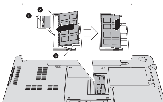
Рисунок 4-14 Установка модуля памяти
