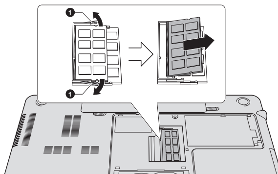
Рисунок 4-16 Удаление модуля памяти
