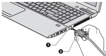
1. Порт для подключения внешнего монитора RGB 2. Кабель монитора
