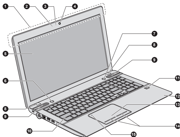
Рисунок 3-6 Вид компьютера спереди с открытой панелью дисплея
