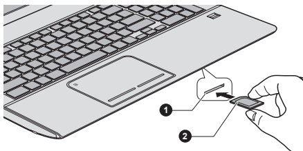
Рисунок 4-18 Установка запоминающего устройства
