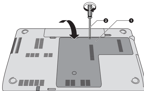
Рисунок 4-15 Установка крышки отсека модулей памяти
