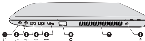
Рисунок 3-3 Правая сторона компьютера
