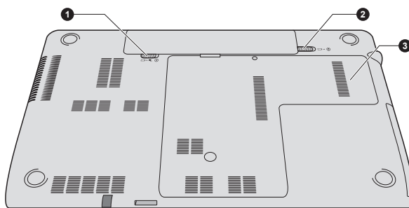
Рисунок 3-5 Вид компьютера снизу
