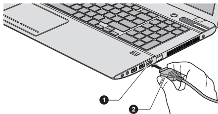
Рисунок 4-20 Подключение к порту выхода HDMI
