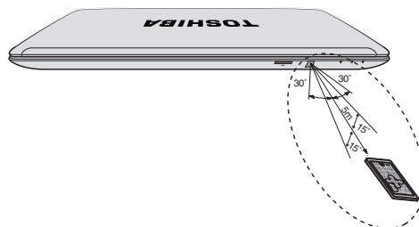
Рисунок 3-8 Радиус действия пульта дистанционного управления
