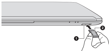
1. Гнездо запоминающего устройства 2. Запоминающее устройство
