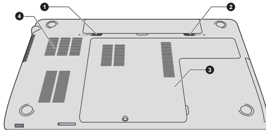
Рисунок 3-5 Вид компьютера снизу
