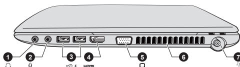
Рисунок 3-3 Правая сторона компьютера
