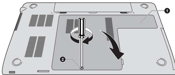
1. Крышка отсека модулей памяти 2. Винт
