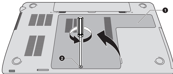
Рисунок 4-13 Снятие крышки отсека модулей памяти
