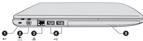
Рисунок 3-2 Левая сторона компьютера
