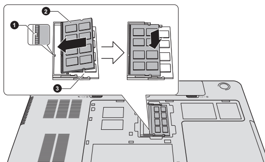
Рисунок 4-14 Установка модуля памяти
