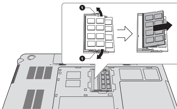
Рисунок 4-16 Удаление модуля памяти
