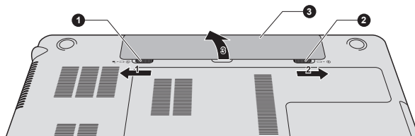
Рисунок 4-11 Высвобождение батарейного источника питания – 1
