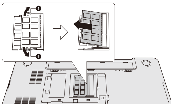
Рисунок 4-15 Удаление модуля памяти
