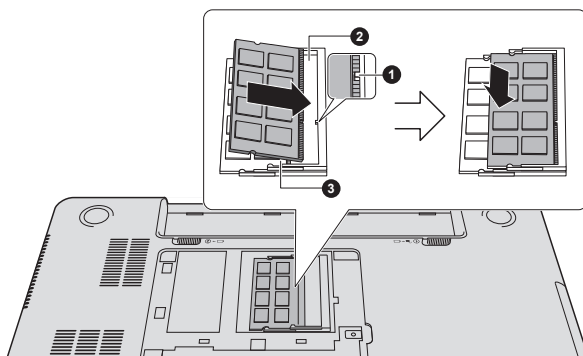
Рисунок 4-13 Установка модуля памяти
