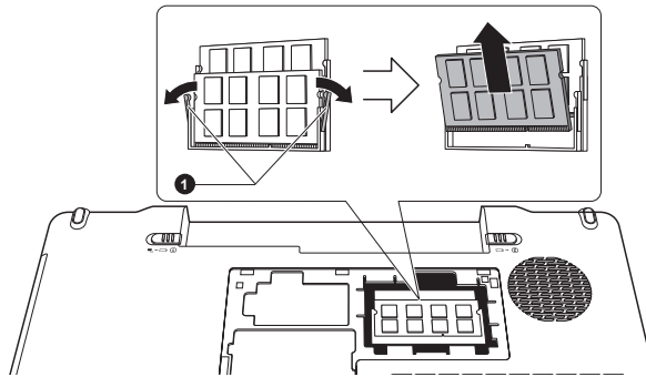
Рисунок 3-14 Удаление модуля памяти
