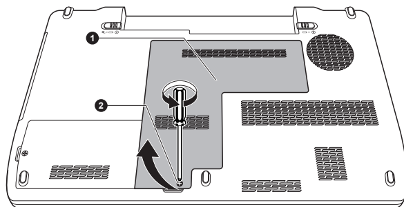
1. Крышка отсека модулей памяти 2. Винт
