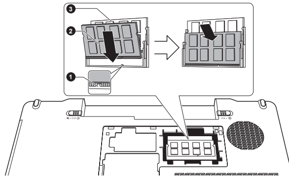
Рисунок 3-12 Установка модуля памяти
