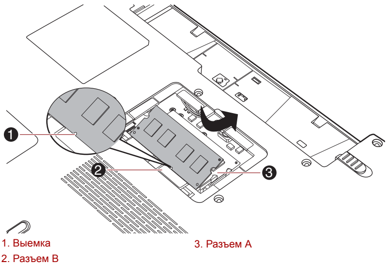
Рисунок 3-4 Установка модуля памяти
