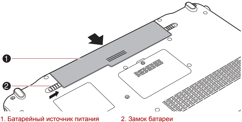
Рисунок 6-2 Закрепление батарейного источника питания
