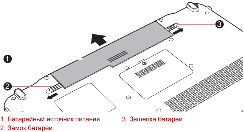
Рисунок 6-1 Высвобождение батарейного источника питания
