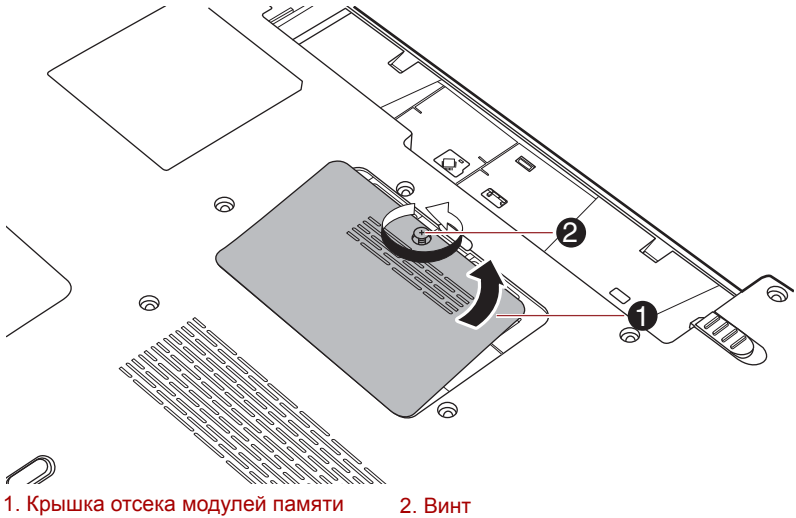
Рисунок 3-3 Снятие крышки отсека модулей памяти
