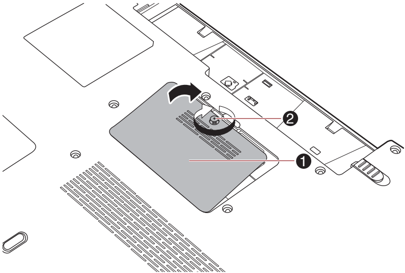
Рисунок 3-5 Установка крышки отсека модулей памяти
