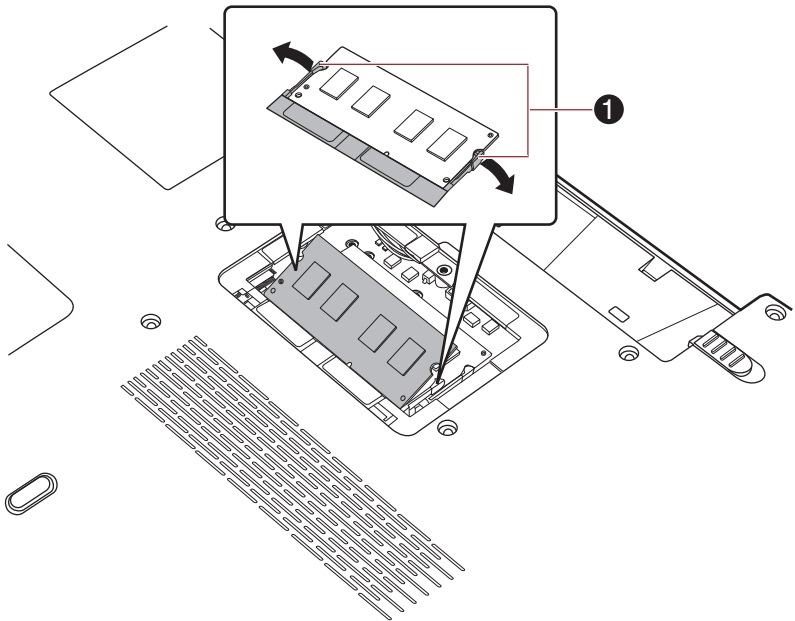
Рисунок 3-6 Удаление модуля памяти
