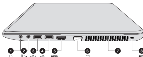
Рисунок 3-3 Правая сторона компьютера
