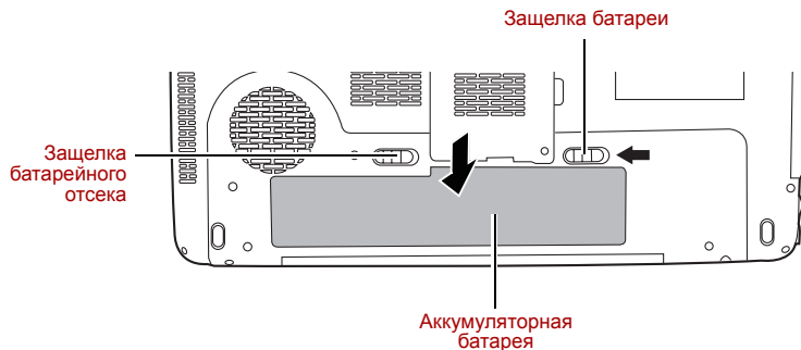
Закрепление аккумуляторной батареи
