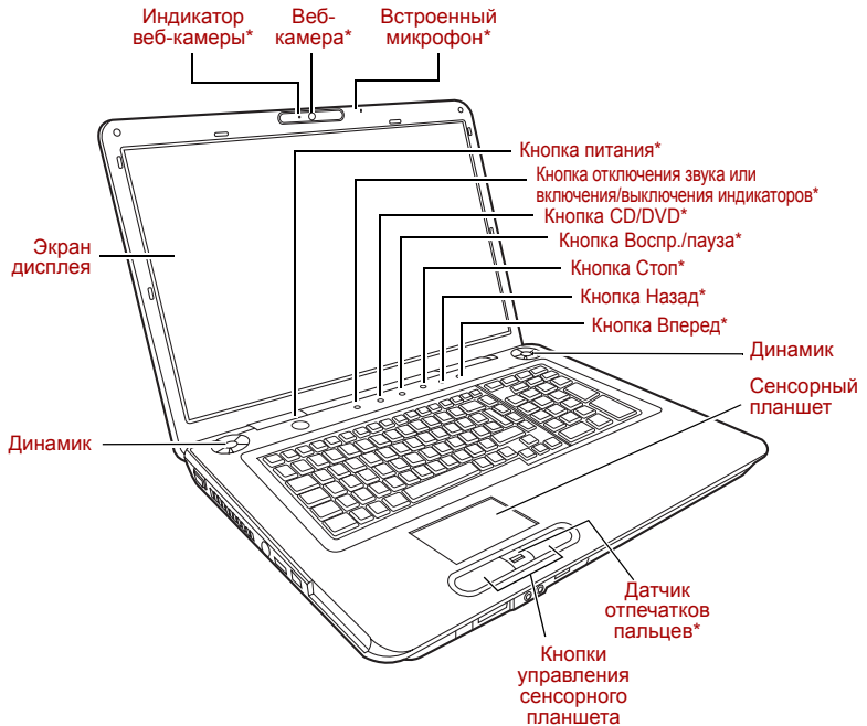
Вид компьютера спереди с открытым дисплеем
