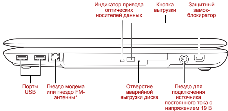
Вид компьютера справа
