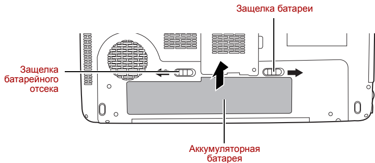
Высвобождение аккумуляторной батареи
