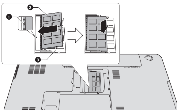
Рисунок 4-12 Установка модуля памяти
