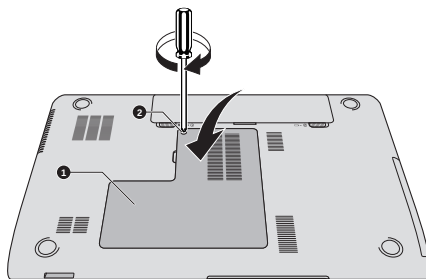
Рисунок 4-13 Установка крышки отсека модулей памяти
