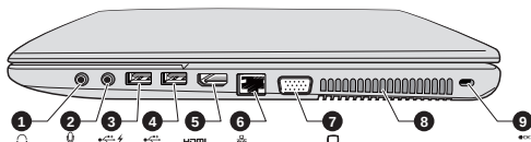
Рисунок 3-3 Правая сторона компьютера
