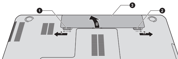
Рисунок 4-10 Высвобождение батарейного источника питания – 2
