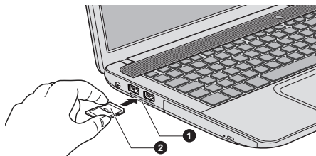
Рисунок 3-11 Установка запоминающего устройства
