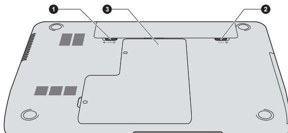
Рисунок 2-5 Вид компьютера снизу
