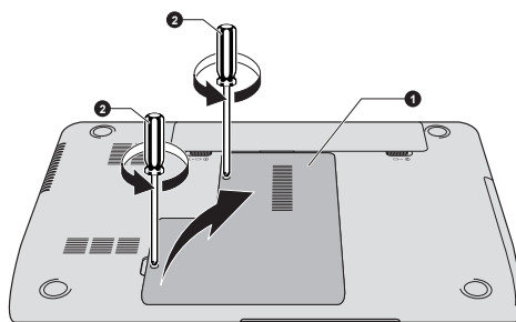
1. Крышка отсека модулей памяти 2. Винты
