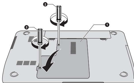
Рисунок 3-14 Установка крышки отсека модулей памяти
