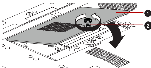
1. Крышка отсека модулей памяти
