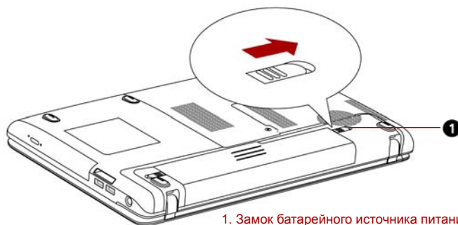
Рисунок 6-1 Сдвиньте блокирующую защелку в разомкнутое положение
