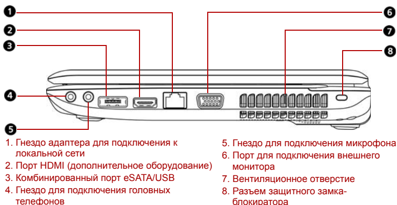
Рисунок 2-3 Правая сторона компьютера
