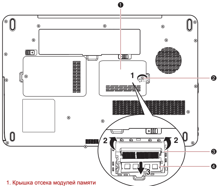
Рисунок 8-2 Снимаем крышку отсека для модулей памяти
