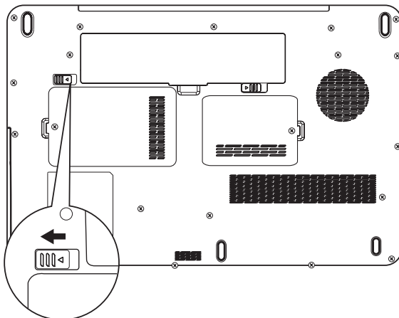
Рисунок 6-1 Высвобождение батарейного источника питания (1)
