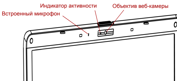
Рисунок 4-14 Веб-камера
