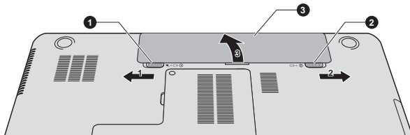
Рисунок 4-9 Высвобождение батарейного источника питания – 1
