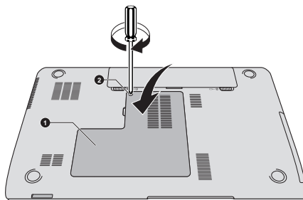
Рисунок 4-13 Установка крышки отсека модулей памяти
