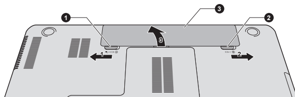
Рисунок 4-10 Высвобождение батарейного источника питания – 2
