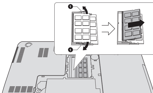
Рисунок 4-14 Удаление модуля памяти
