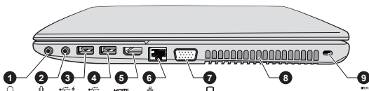
Рисунок 3-3 Правая сторона компьютера
