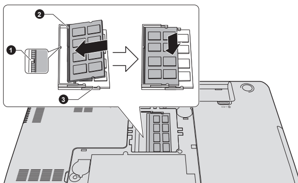
Рисунок 4-12 Установка модуля памяти
